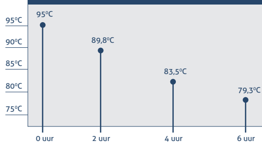
Isolatiewaarde Gastroline isoleerkan
